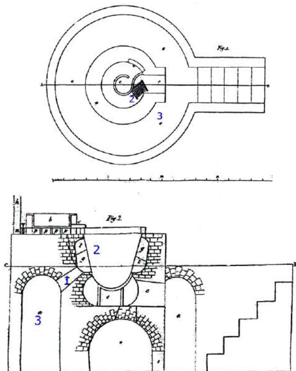
Figura 12. Horno del interior de los cuartos cuajadores. Existía una especie de cenicero (1) donde eliminar las cenizas de la caldera, situada sobre la rejilla de hierro donde se colocaba la leña (2). El claustrillo era una especie de pasaje interior donde se encendía el fuego a través de la propia boca encima del cenicero. Modificado de Martínez Rueda (1833).
