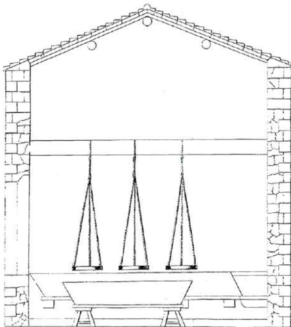
Figura 21. Aspecto lateral de un cuarto graneador con la viga de la que cuelgan los tres arrompedores utilizados para el graneo. Modificado de Martínez Rueda (1833).
