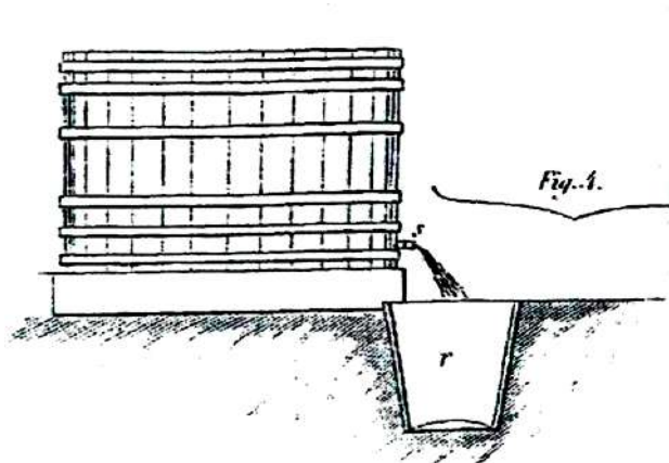
Figura 17. Esquema original de un botazo de lavado. En él se introducían las arenillas (salitre sencillo machacado), que se lavaban y se extraía el salitre afinado. Los restos de impurezas quedaban depositados bajo la espita, entre capas de madera y esparto. Modificado de Martínez Rueda (1833).
