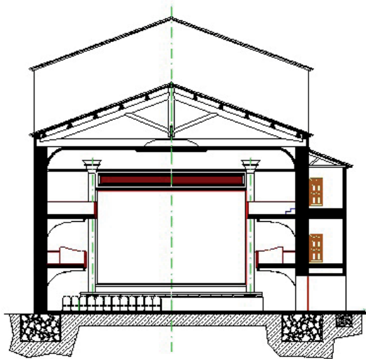
Teatro-Cine CRISFEL Alcázar de San Juan (C.R.) SECCIÓN, B-B' (Transversal) ESO BIARDO Dibujado: Alberto OENJOR OREA Marzo, 2010. Fuera de Escala
