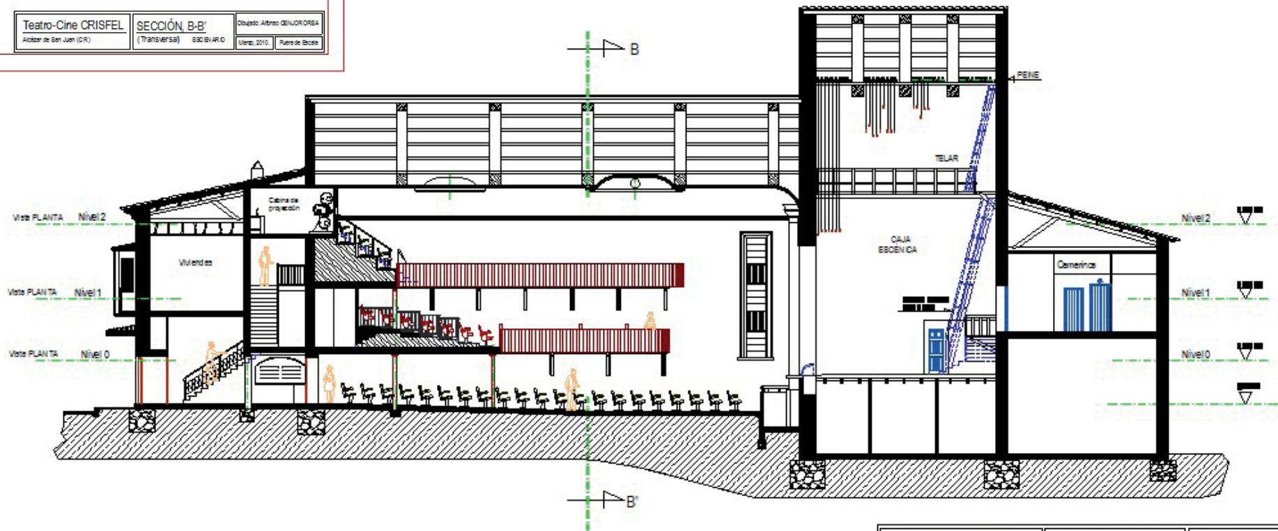
Teatro-Cine CRISFEL Alcázar de San Juan (C.R.) SECCIÓN, A-A' (Longitudinal) Dibujado: Alberto OENJOR OREA Marzo, 2010. Fuera de Escala
